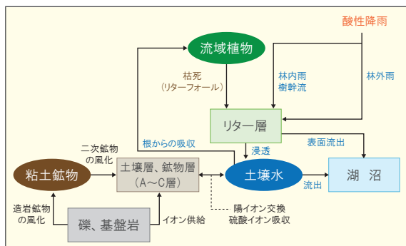
図1 集水域による酸性雨の緩衝作用とモデル化
