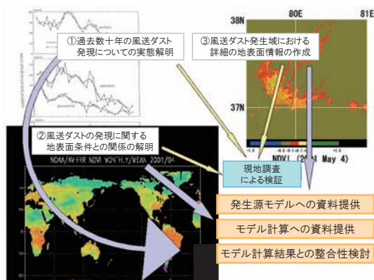
図2 風送ダストの変動とその機構解明に関する研究の流れ
