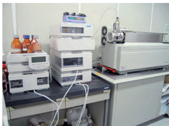
写真1 液体クロマトグラフ質量分析計(LC/MS/MS)
