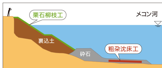
図2 パイロット護岸工事の断面図
