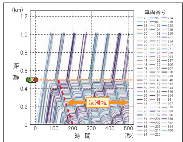
図4 交差点における車両の挙動
