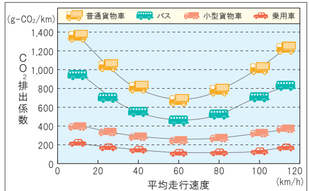
図1 CO 2 排出係数と平均走行速度の関係 3)
