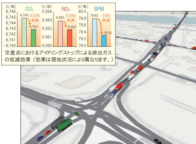
図3 交通マイクロシミュレータを用いたCO 2 、NO 2 、SPM排出量の計測
