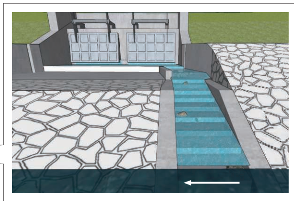
対象魚種の遡上を可能とする階段式魚道の検討 (遡上能力を考慮した水理計算結果による設計)
